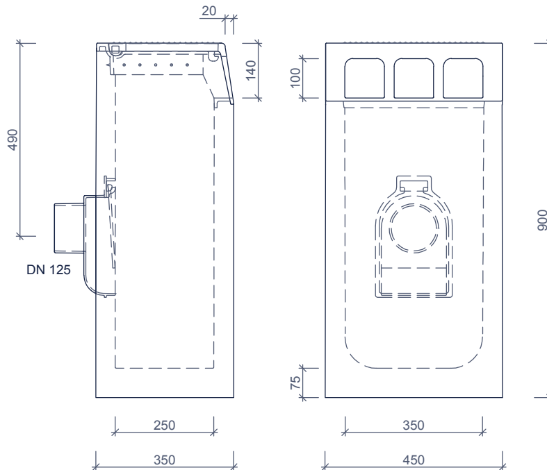
zijaanzichten vues de côté
